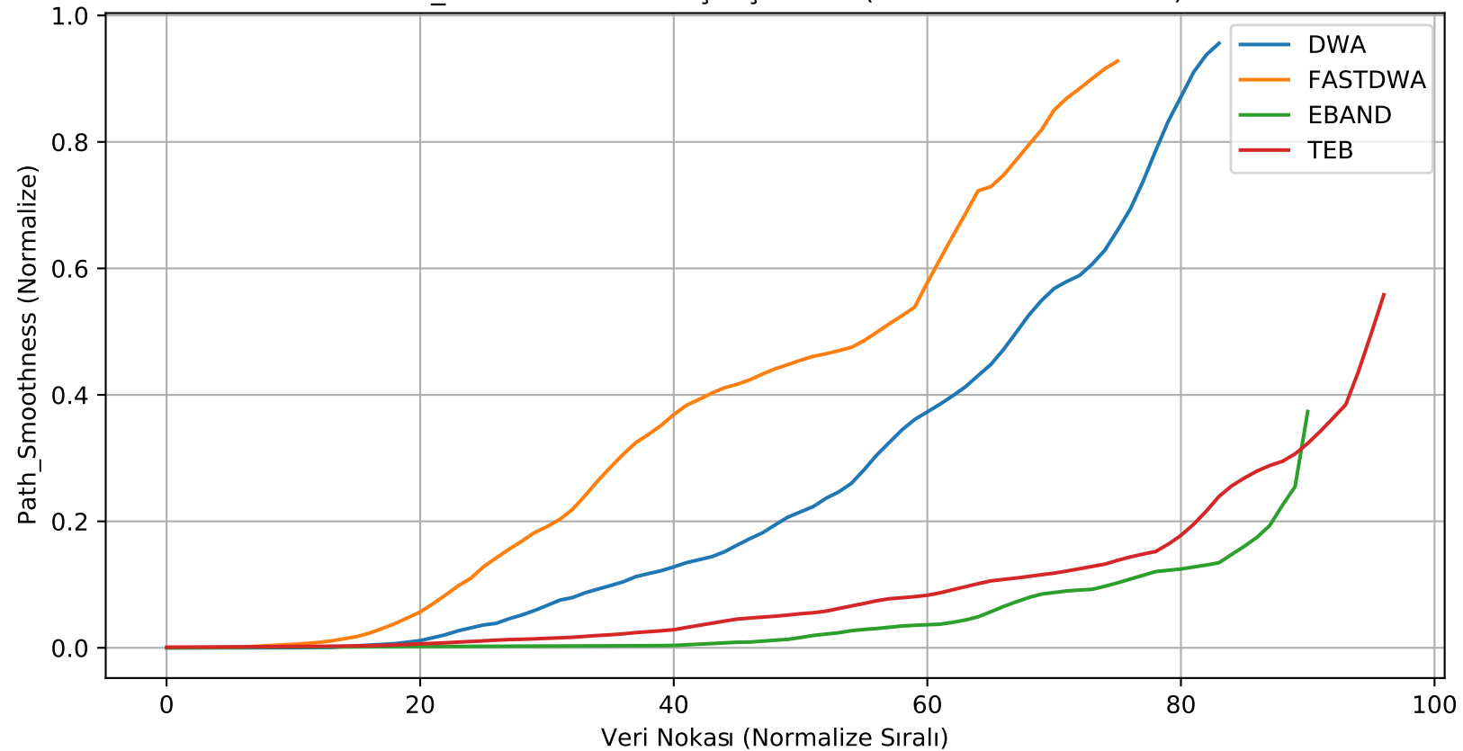
Path_Smoothness - Karşılaştırmalı (Normalize + Smooth)
